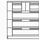
OH: 825 OW: 760 OD: 480
